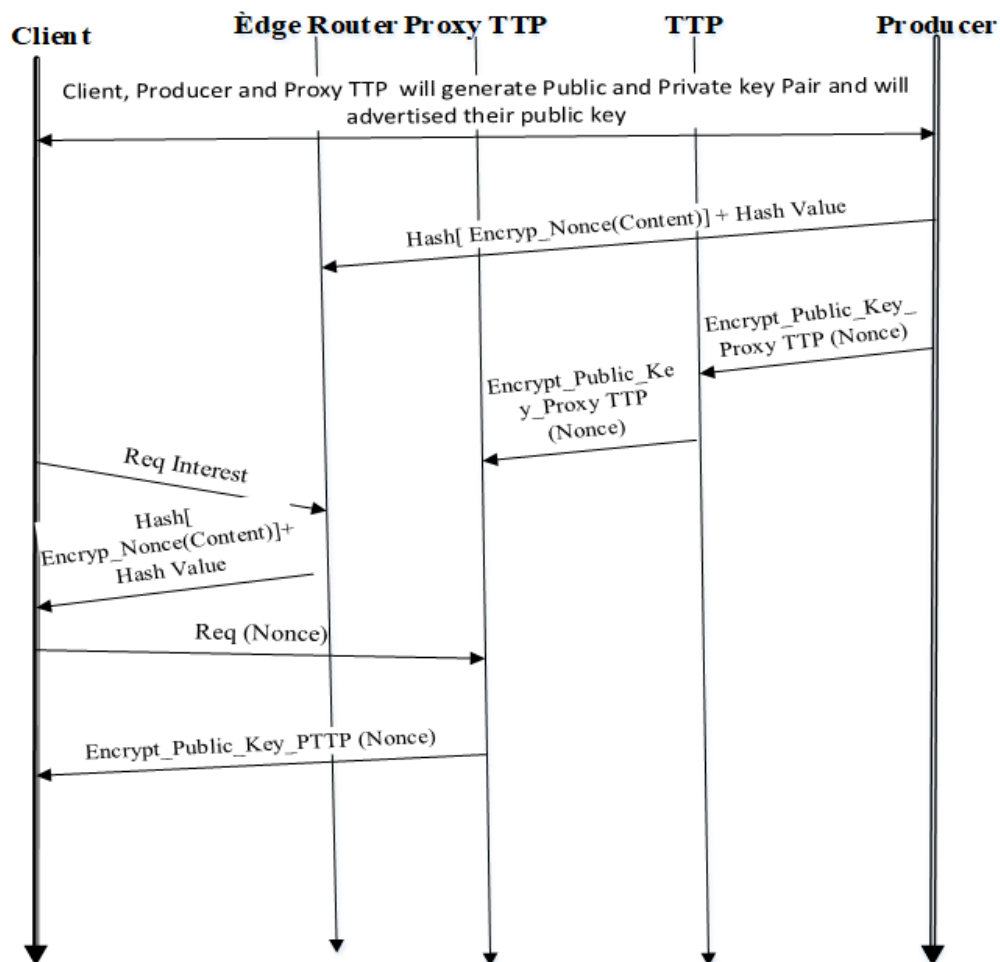
Figure 3.4 Timeline data flow diagram of ICN using DSAC with TTP .
