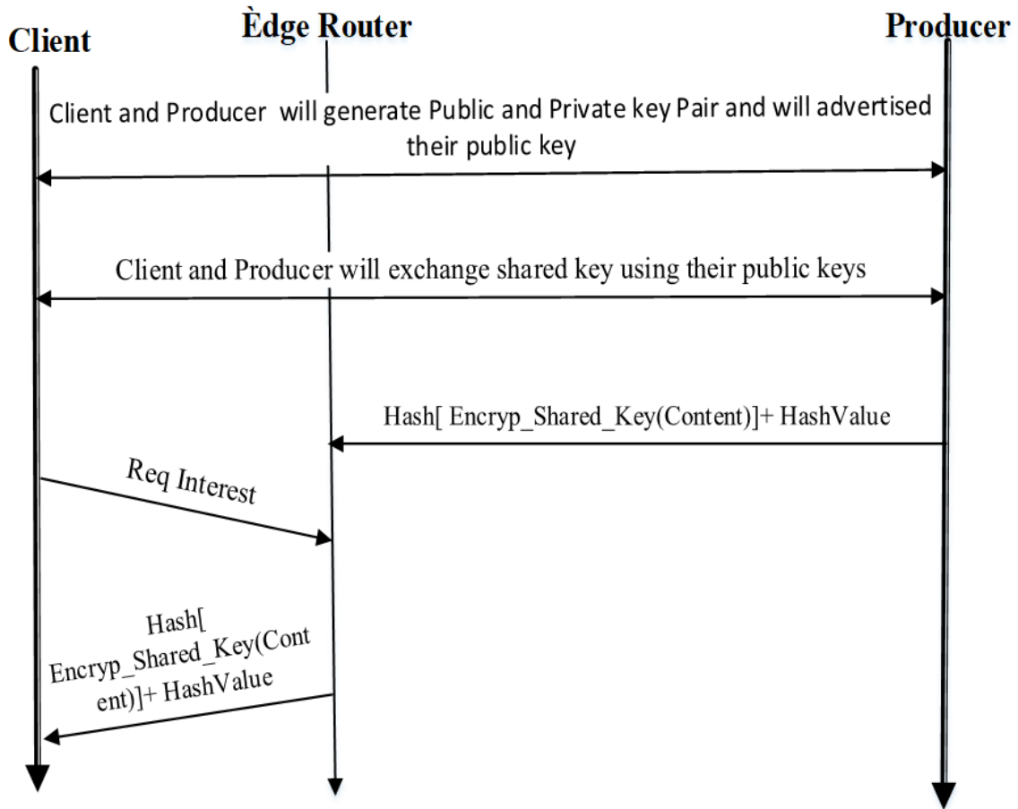
Figure 3.3 Timeline data flow diagram of ICN using DSAC without TTP.
